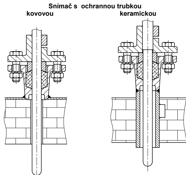
OBRÁZEK 2 - PŘÍKLADY MONTÁŽE UPEVNĚVACÍCH PŘÍRUB PRO TYČOVÉ SNÍMAČE S KOVOVOU A KERAMICKOU OCHRANNOU TRUBKOU
