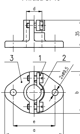
Příruba UP18
