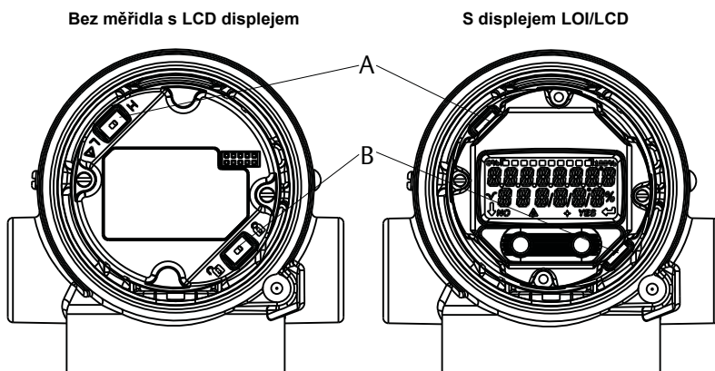
Obrázek 8. Umístění propojek na desce elektroniky převodníku
