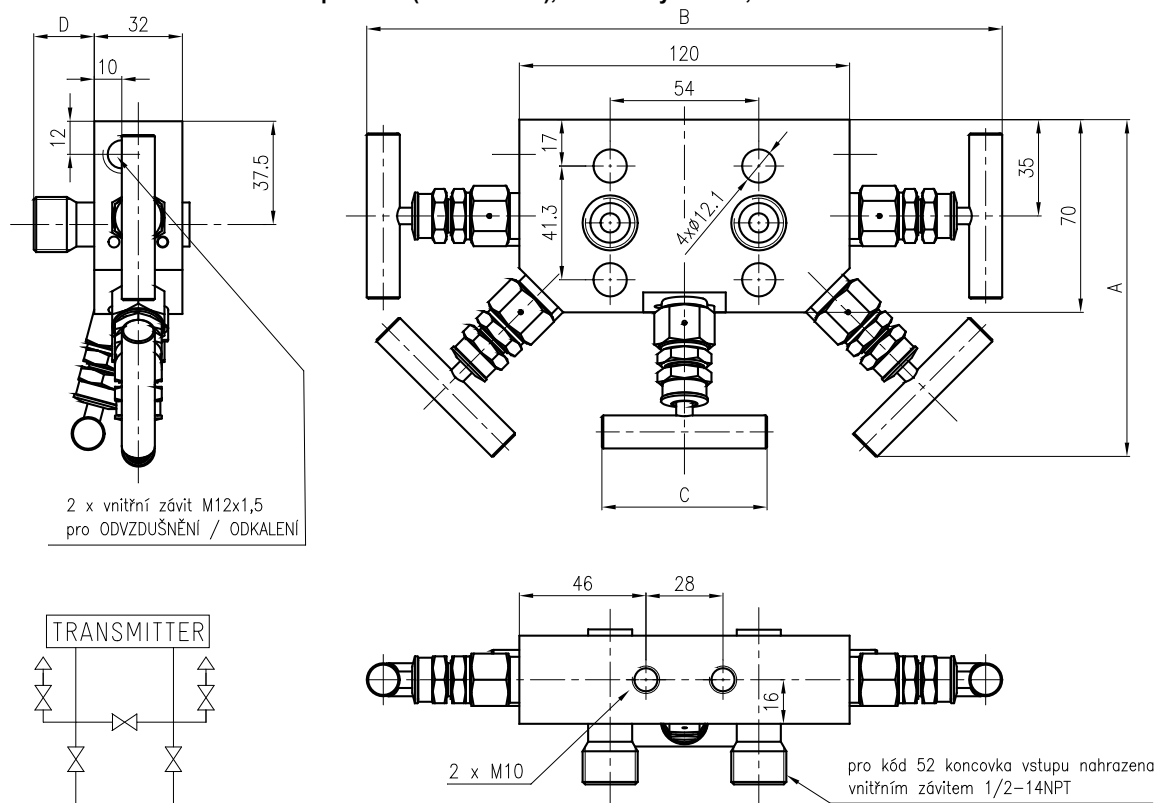
Obrázek 10 - Pěticestná ventilová souprava (964 25.. AS1), rozměrový nákres, schéma
