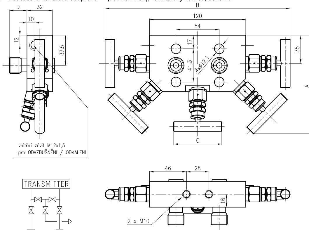
Obrázek 11 - Pěticestná ventilová souprava (964 25.. AS2), rozměrový nákres, schéma
