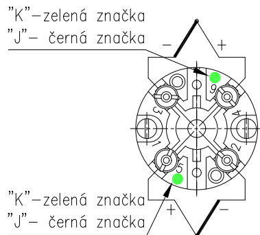
OBRÁZEK 3 - PŘÍKLAD PROVOZNÍHO ZAPOJENÍ SNÍMAČE TEPLoty S PŘEVODNÍKEM VE SMYČCE 4 - 20 mA
