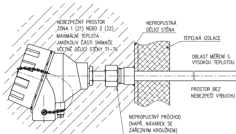
OBRÁZEK 5 - PŘÍKLAD MONTÁŽE SNÍMAČŮ TEPLoty Ex d S KOVOVOU OCHRANNOU TRUBKOU (pro případ, kdy je požadována horní mez rozsahu měření vyšší než požadovaná teplotní třída)
