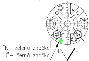
OBRÁZEK 2 - SCHÉMA ZAPOJENÍ SNÍMAČŮ TEPLoty bez převodníku s termočlánkem jednoduchým
