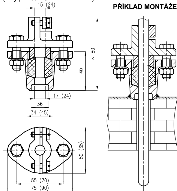
PŘÍKLAD MONTÁŽE
