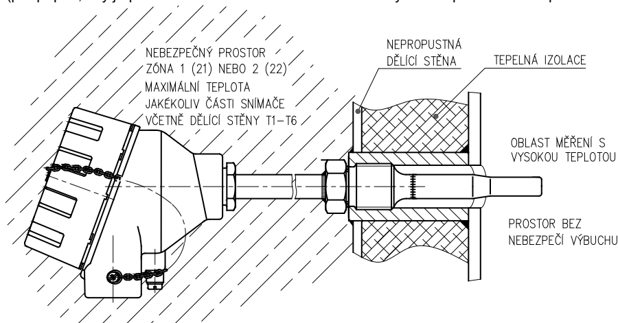
OBRÁZEK 6 - OZNAČENÍ NEVÝBUŠNOSTI
