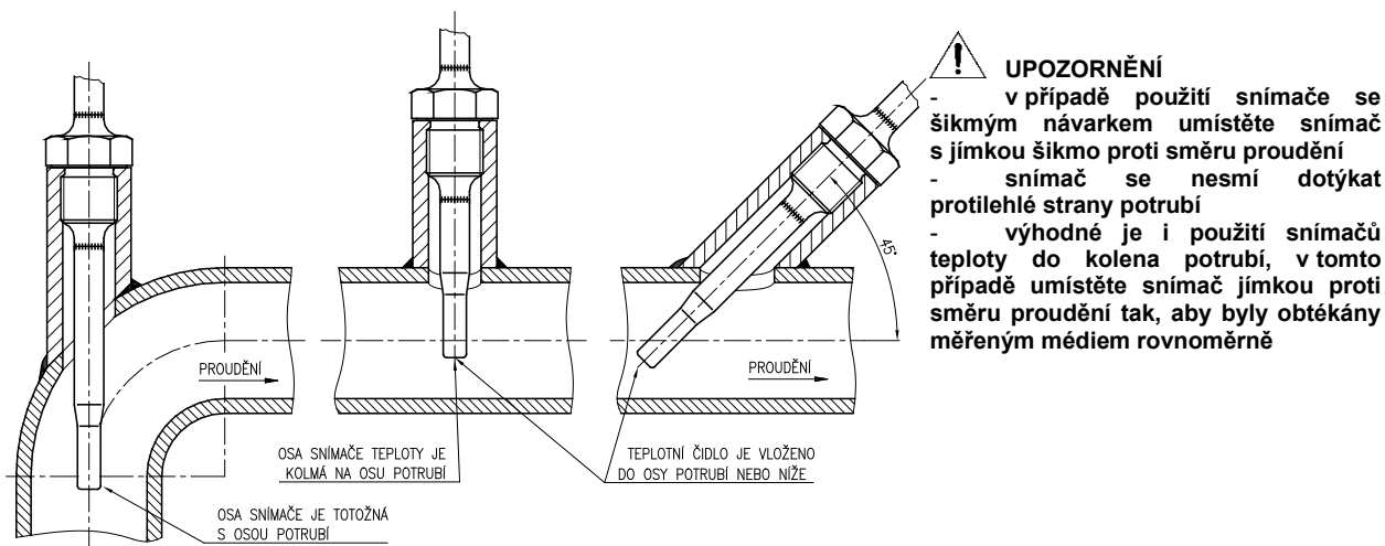
OBRÁZEK 5 - PŘÍKLAD MONTÁŽE SNÍMAČŮ TEPLoty Ex d s JÍMKOU DIN
