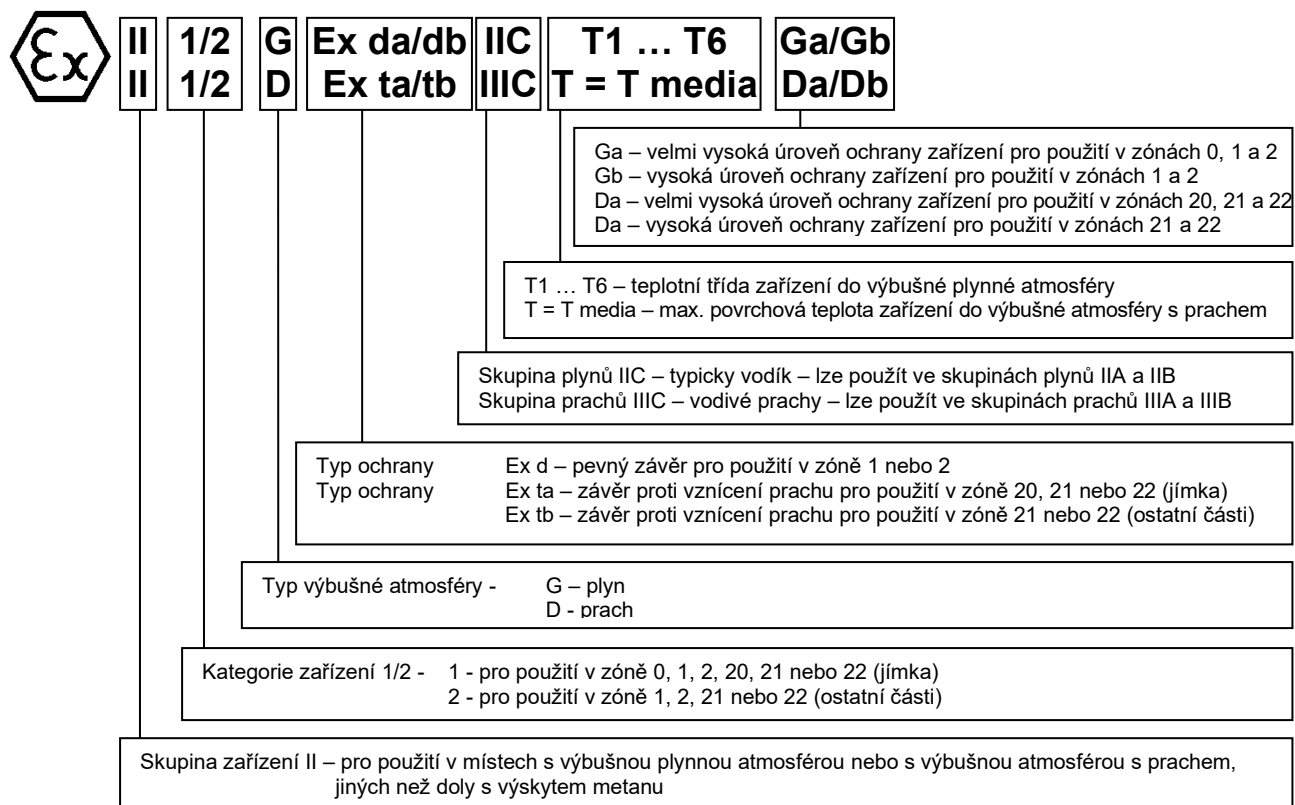
OBRÁZEK 5 - OZNAČENÍ NEVÝBUŠNOSTI
