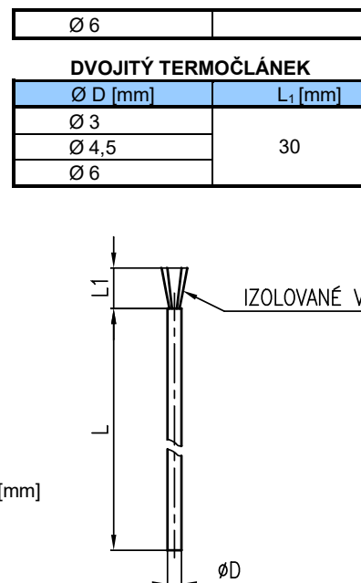
OBRÁZEK 4 ROZMĚROVÝ NÁKRES – PROVEDENÍ C s přechodkou a kompenzačním vedením
