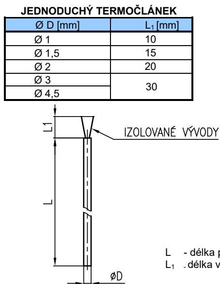
OBRÁZEK 2 - ROZMĚROVÝ NÁKRES – PROVEDENÍ A s volnými vývody větví (standardní provedení)
