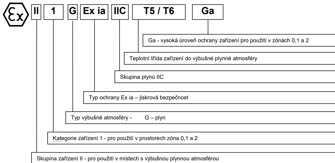
OBRÁZEK 10 - OZNAČENÍ JISKROVÉ BEZPEČNOSTI
