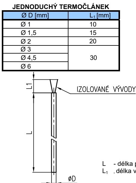
OBRÁZEK 2 - ROZMĚROVÝ NÁKRES - PROVEDENÍ A s volnými vývody větví (standardní provedení)
