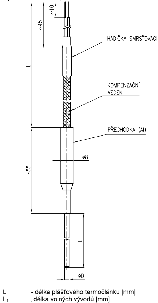
OBRÁZEK 4 ROZMĚROVÝ NÁKRES - PROVEDENÍ C s přechodkou a kompenzačním vedením
