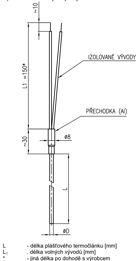
OBRÁZEK 3 ROZMĚROVÝ NÁKRES - PROVEDENÍ B s přechodkou a volnými vývody větvi
