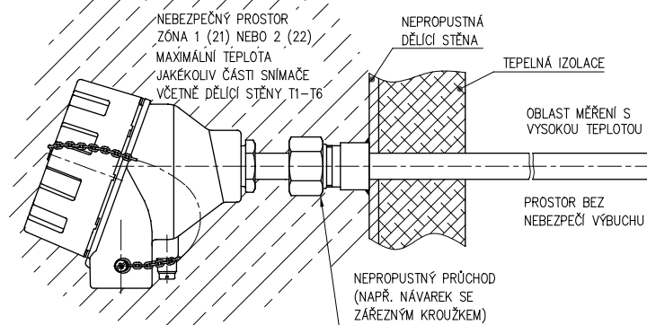
OBRÁZEK 5 - PŘÍKLAD MONTÁŽE SNÍMAČŮ TEPLOTY Ex d S KOVOVOU OCHRANNOU TRUBKOU
