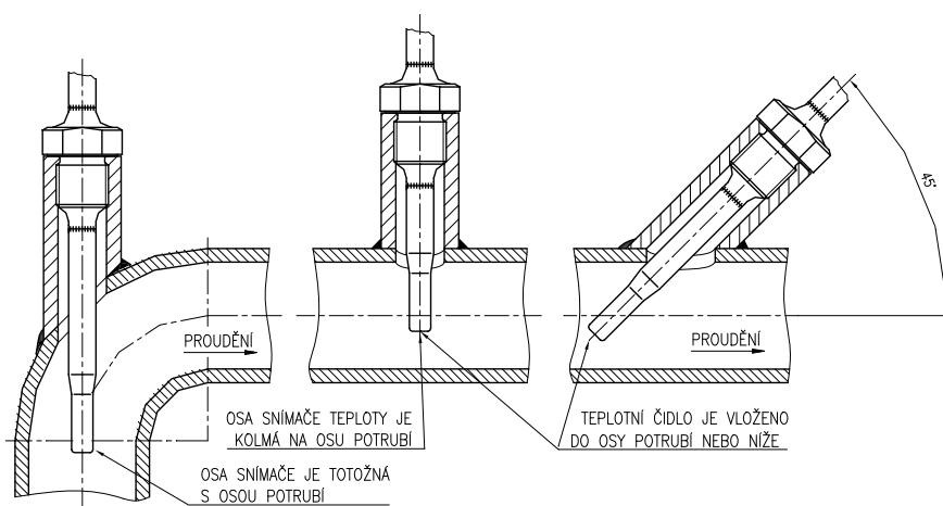
OBRÁZEK 4 - PŘÍKLADY MONTÁŽE PŘÍMÝCH A ŠIKMÝCH NÁVARKŮ DLE ČSN EN 1434-2+A1
