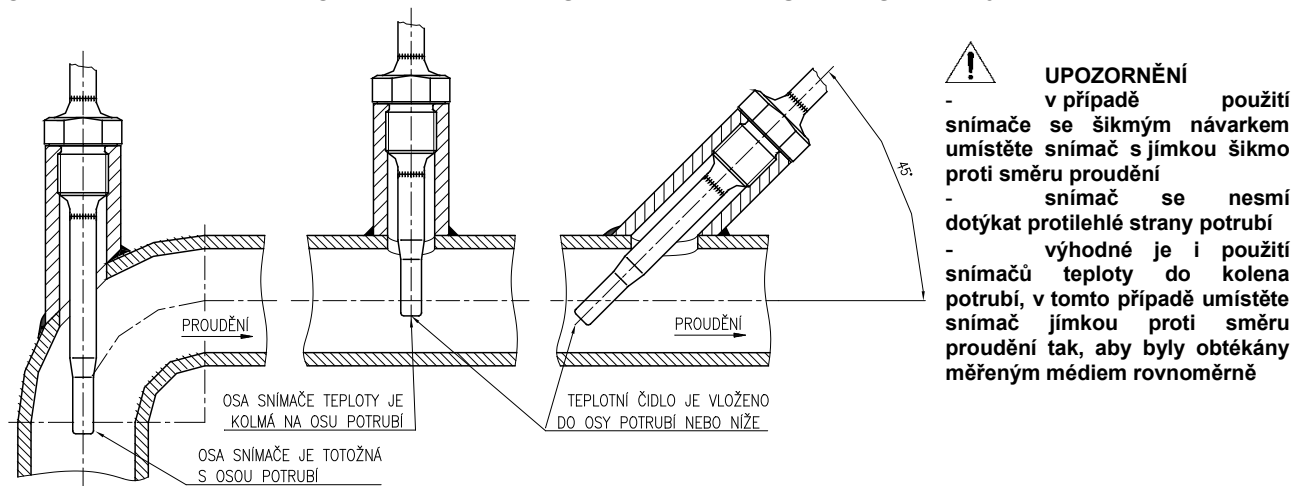
OBRÁZEK 4 - PŘÍKLADY MONTÁŽE PŘÍMÝCH A ŠIKMÝCH NÁVARKŮ DLE ČSN EN 1434-2
