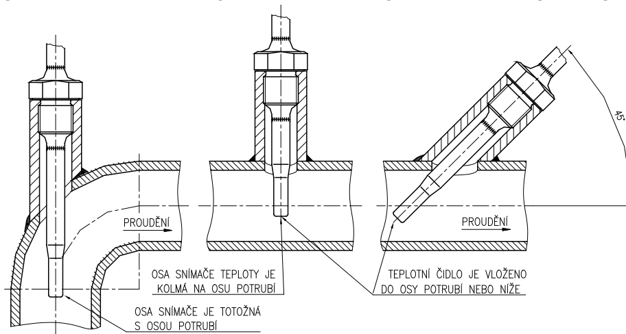
OBRÁZEK 4 - PŘÍKLADY MONTÁŽE PŘÍMÝCH A ŠIKMÝCH NÁVARKŮ DLE ČSN EN 1434-2
