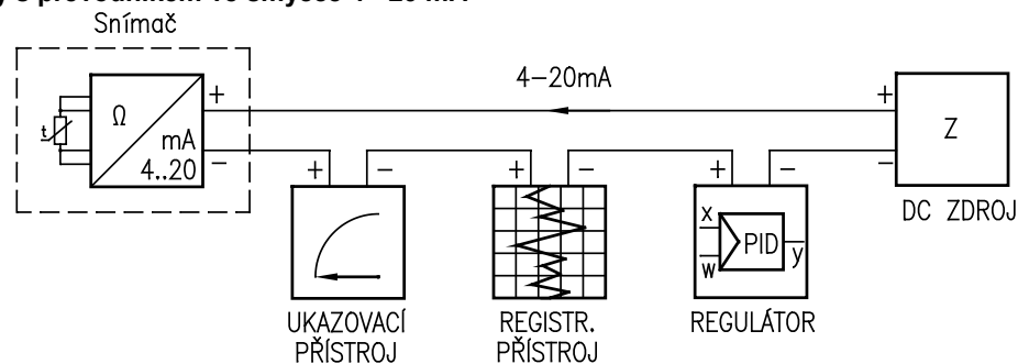
OBRÁZEK 3 - VZOR PROVOZNÍHO ZAPOJENÍ snímače teploty s převodníkem ve smyčce 4 - 20 mA
