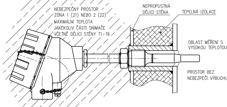
OBRÁZEK 3 - PŘÍKLAD MONTÁŽE SNÍMAČŮ TEPLoty Ex d S JÍMKOU DIN
