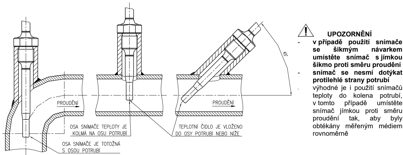
OBRÁZEK 2 - PŘÍKLADY MONTÁŽE PŘÍMÝCH A ŠIKMÝCH NÁVARKŮ DLE ČSN EN 1434-2
