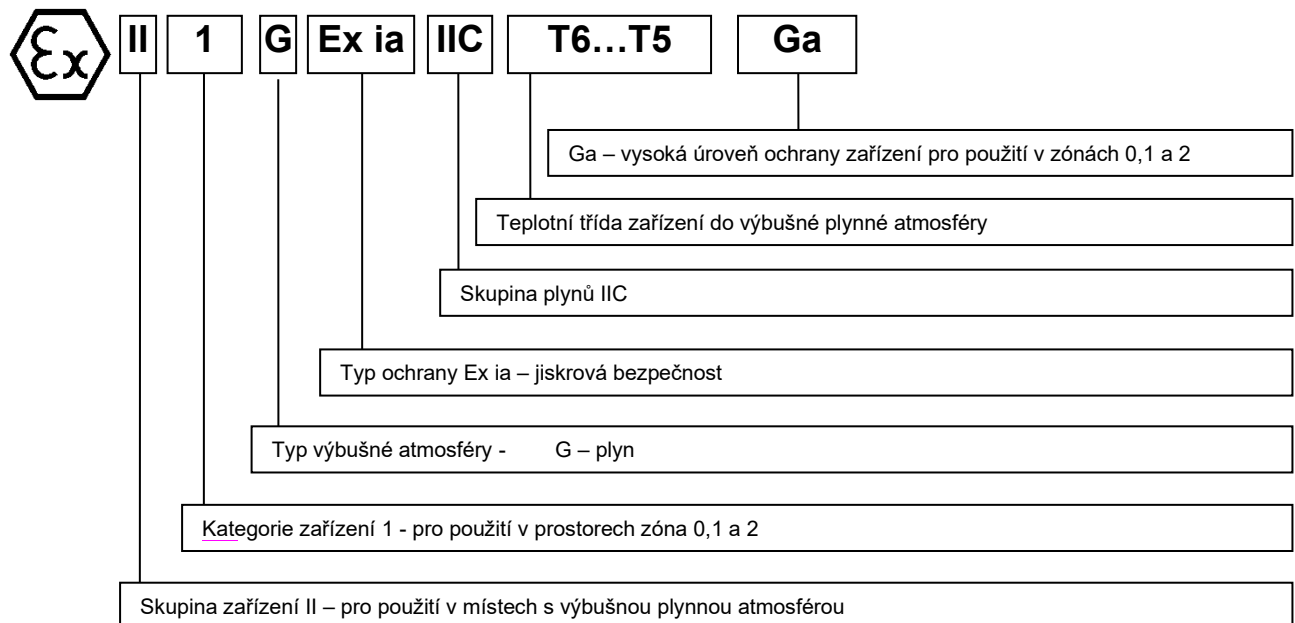
OBRÁZEK 5 - OZNAČENÍ JISKROVÉ BEZPEČNOSTI
