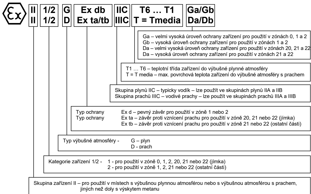
OBRÁZEK 4 - OZNAČENÍ NEVÝBUŠNOSTI
