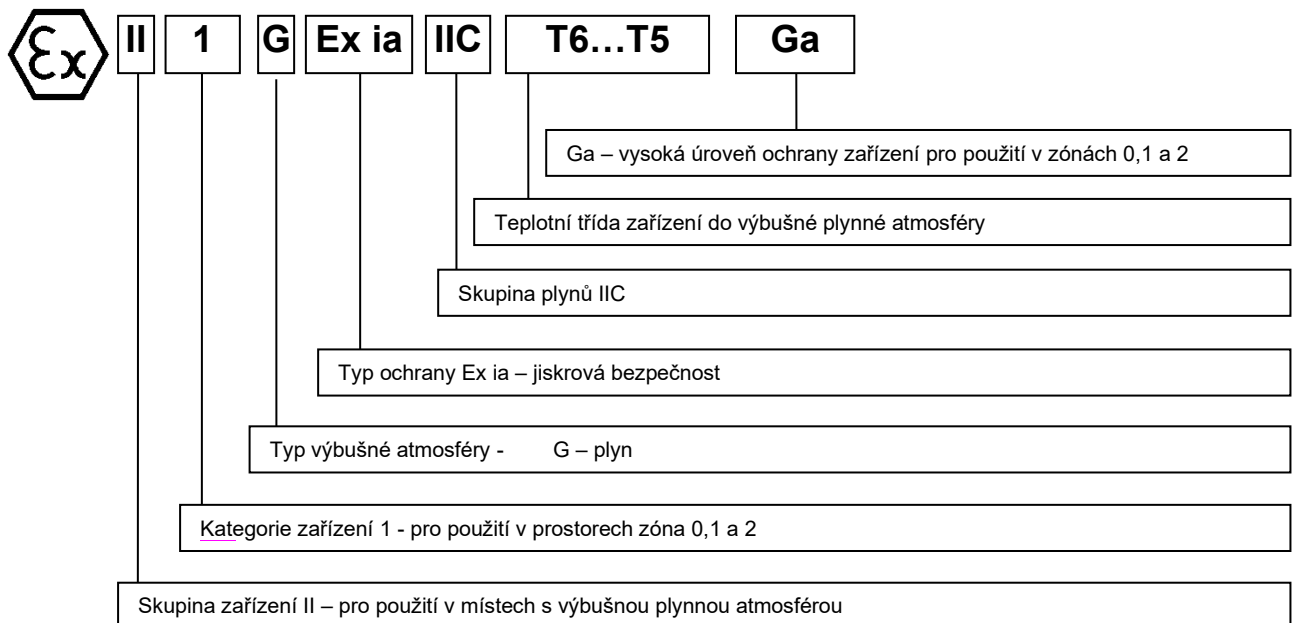
OBRÁZEK 5 - OZNAČENÍ JISKROVÉ BEZPEČNOSTI
