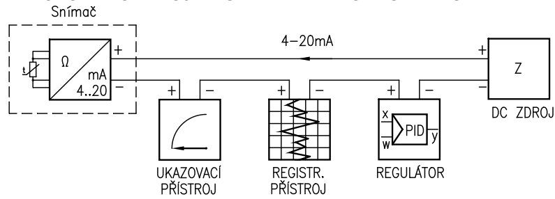
OBRÁZEK 3- PŘÍKLAD PROVOZNIHO ZAPOJENÍ SNÍMAČE TEPLoty S PŘEVODNÍKEM VE SMYČCE 4 - 20 MA
