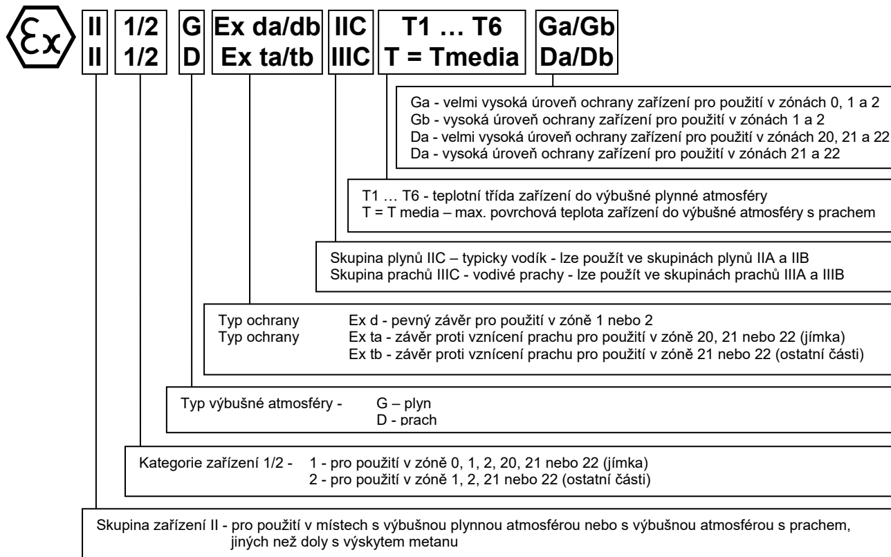
OBRÁZEK 4 - OZNAČENÍ NEVÝBUŠNOSTI
