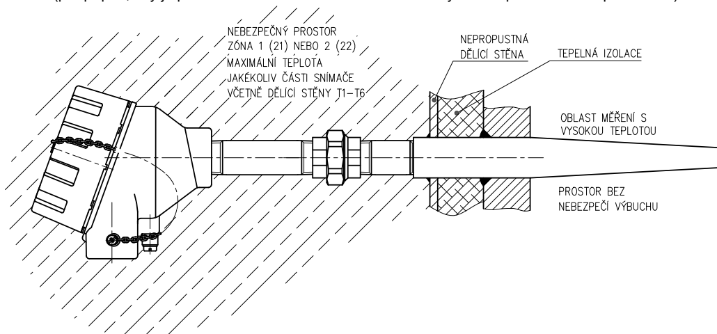
OBRÁZEK 6 - PŘÍKLAD MONTÁŽE SNÍMAČŮ TEPLoty Ex d DO JÍMKY DIN
