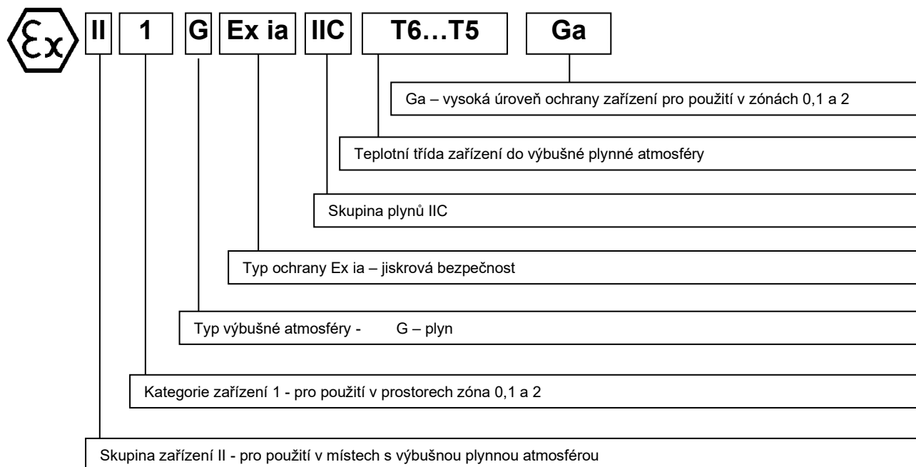
OBRÁZEK 4 - OZNAČENÍ JISKROVÉ BEZPEČNOSTI
