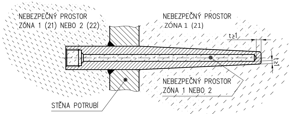
OBRÁZEK 5 – JÍMKA PRO SNÍMAČ TEPLoty Ex d PRO ZÓNU 1 (21)
