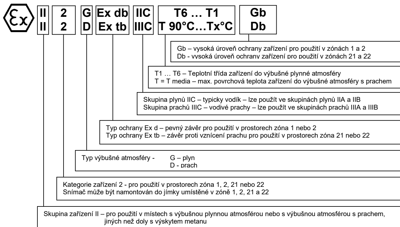
OBRÁZEK 5 - OZNAČENÍ NEVÝBUŠNOSTI
