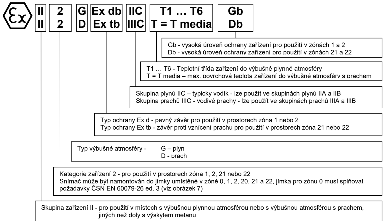
OBRÁZEK 5 - OZNAČENÍ NEVÝBUŠNOSTI
