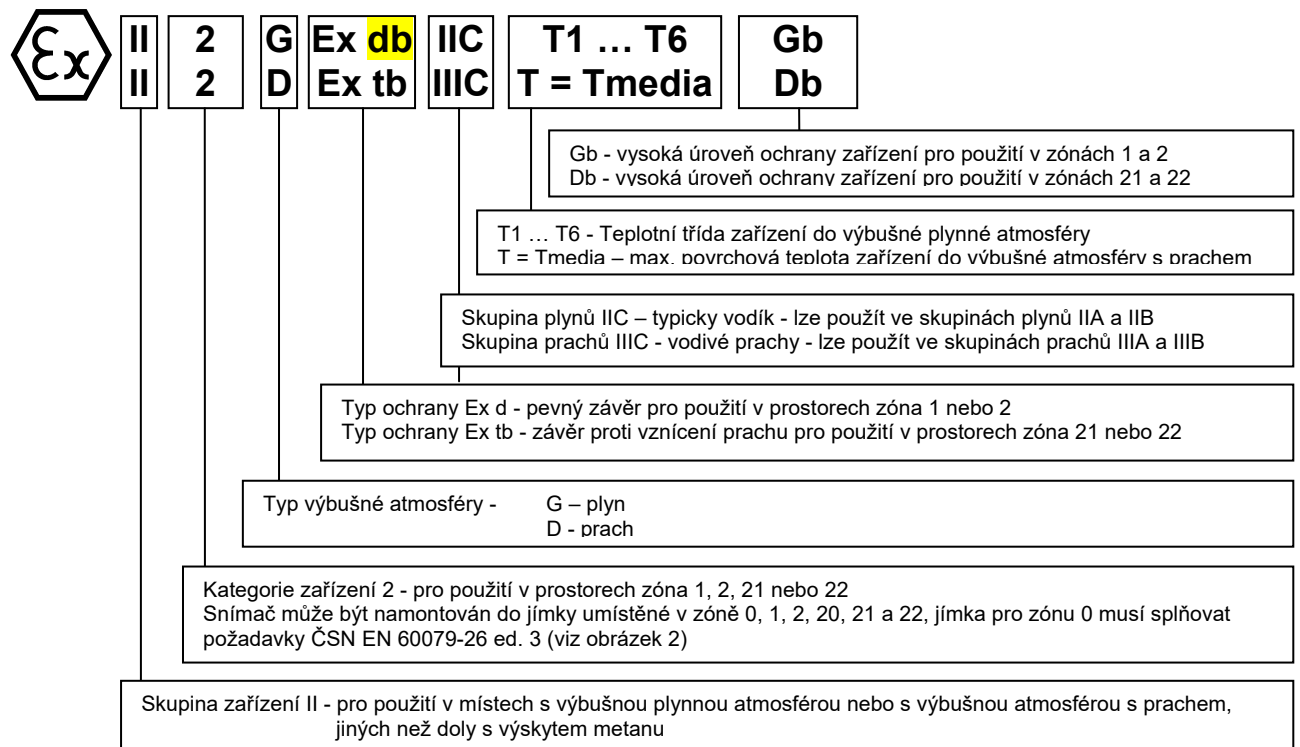
OBRÁZEK 1 - OZNAČENÍ NEVÝBUŠNOSTI
