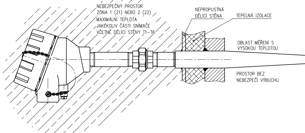
OBRÁZEK 3 - PŘÍKLAD MONTÁŽE SNÍMAČŮ TEPLoty Ex d DO JÍMKY DIN
