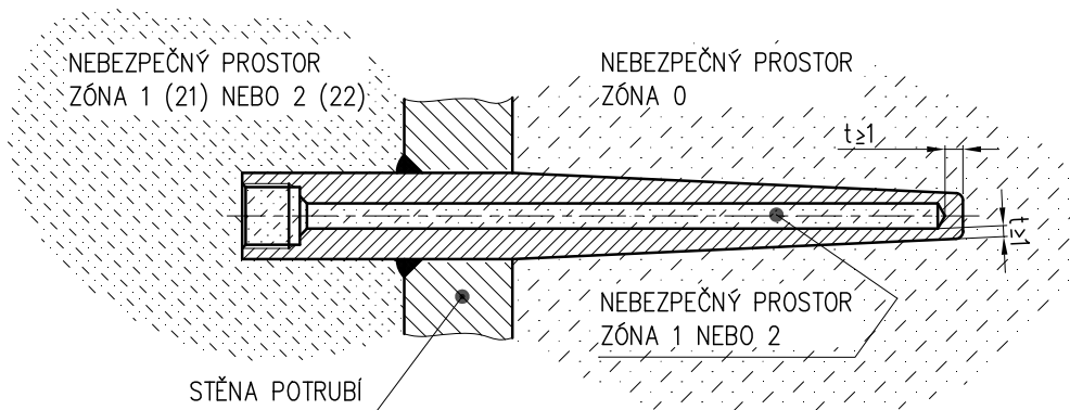
OBRÁZEK 2 – JÍMKA PRO SNÍMAČ TEPLoty Ex d PRO ZÓNU 0 (dle ČSN EN 60079-26 ed. 3)
