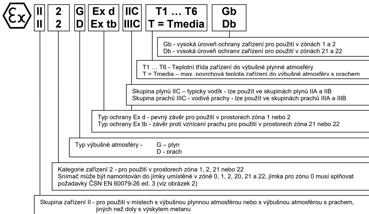
OBRÁZEK 1 - OZNAČENÍ NEVÝBUŠNOSTI
