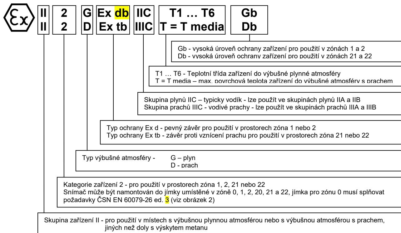
OBRÁZEK 1 - OZNAČENÍ NEVÝBUŠNOSTI
