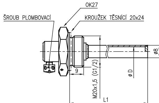
OBRÁZEK 2 – JÍMKA 991 101 A 102
