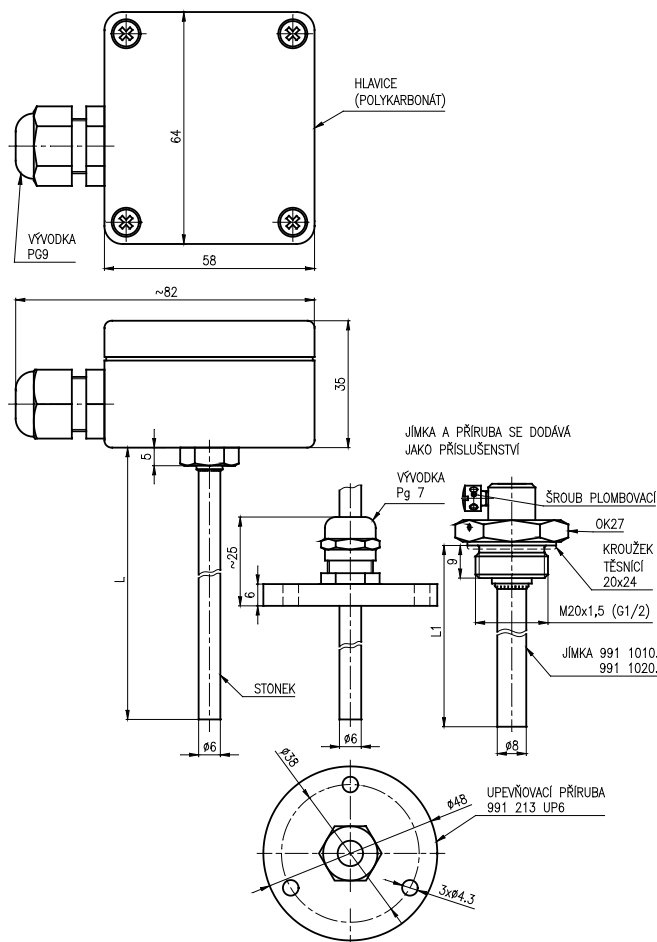
OBRÁZEK 1 – ROZMĚROVÝ NÁKRES
