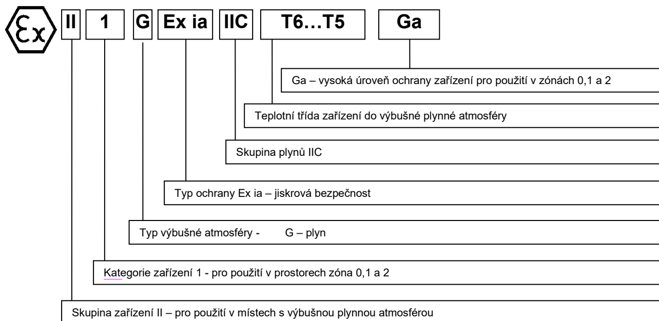
OBRÁZEK 3 - OZNAČENÍ JISKROVÉ BEZPEČNOSTI
