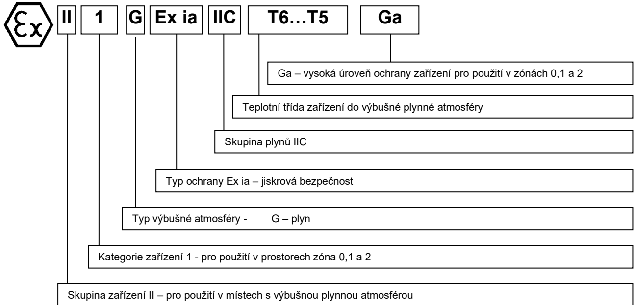
OBRÁZEK 3 - OZNAČENÍ JISKROVÉ BEZPEČNOSTI
