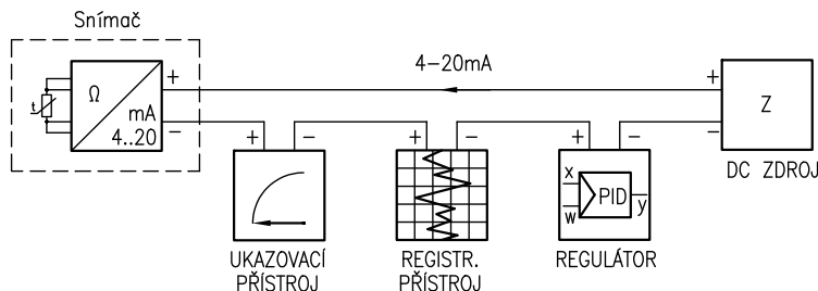
OBRÁZEK 2- PŘÍKLAD PROVOZNIHO ZAPOJENÍ SNÍMAČE TEPLoty S PŘEVODNÍKEM VE SMYČCE 4 - 20 MA
