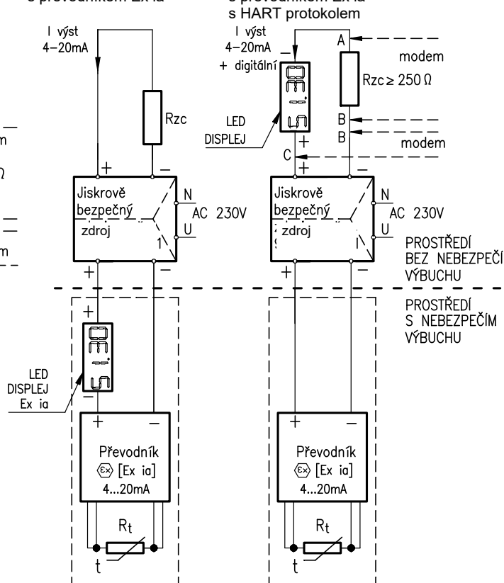
OBRÁZEK 5- PŘÍKLAD PROVOZNÍHO ZAPOJENÍ SNÍMAČE TEPLoty S PŘEVODNÍKEM VE SMYČCE 4 - 20 mA
