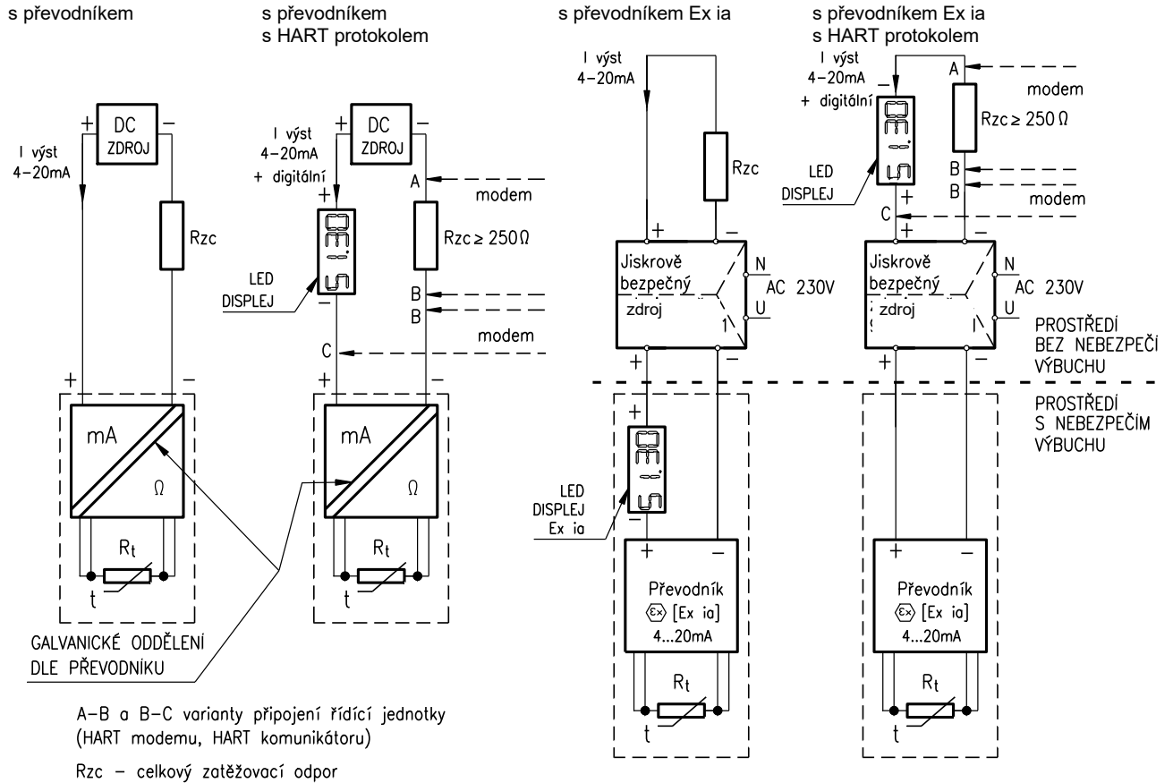
OBRAZEK 6- PŘÍKLAD PROVOZNIHO ZAPOJENÍ SNÍMAČE TEPLoty S PŘEVODNÍKEM VE SMYČCE 4 - 20 mA
