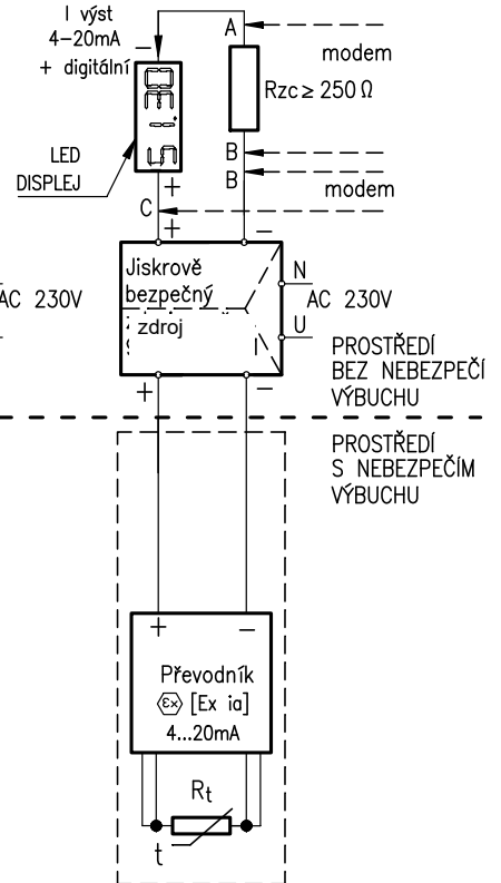
OBRAZEK 6- PŘÍKLAD PROVOZNIHO ZAPOJENÍ SNÍMAČE TEPLoty S PŘEVODNÍKEM VE SMYČCE 4 - 20 mA
