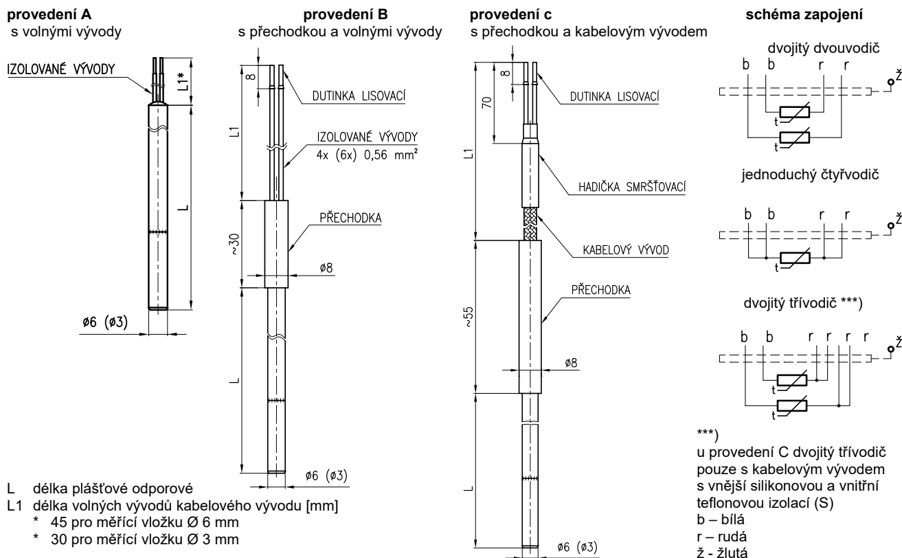
OBRÁZEK 2 - ROZMĚROVÝ NÁKRES
