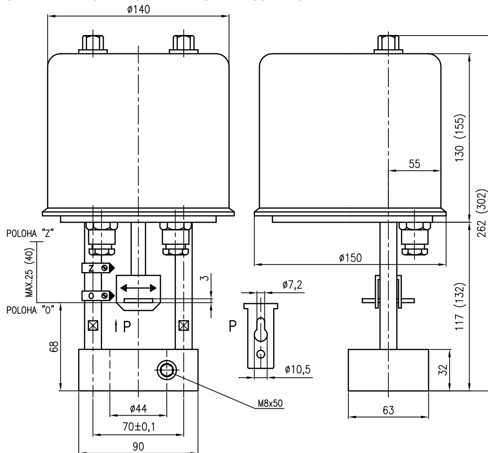
OBRÁZEK 5 - ROZMĚROVÝ NÁKRES – PŘIPOJENÍ P9
