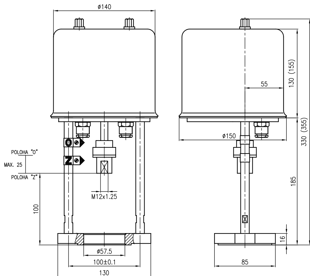
OBRÁZEK 6 - ROZMĚROVÝ NÁKRES – PŘIPOJENÍ P10
