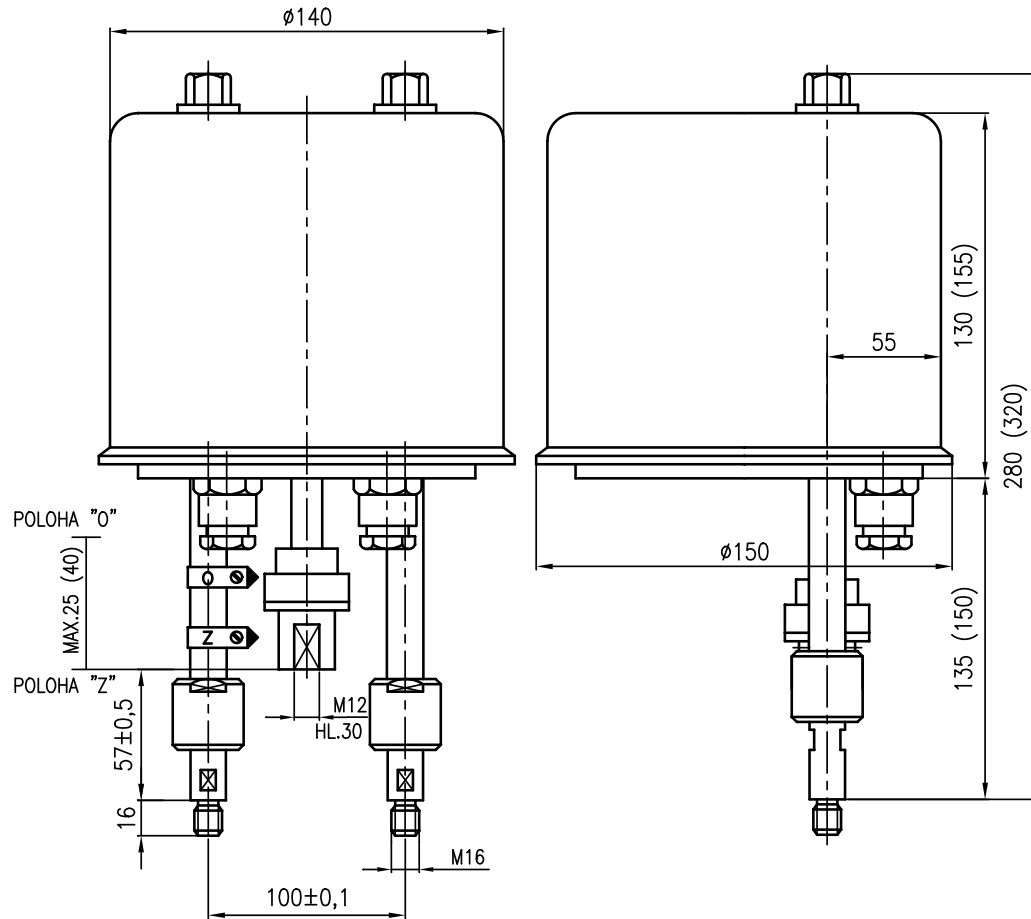
OBRÁZEK 3 - ROZMĚROVÝ NÁKRES – PŘIPOJENÍ P4
