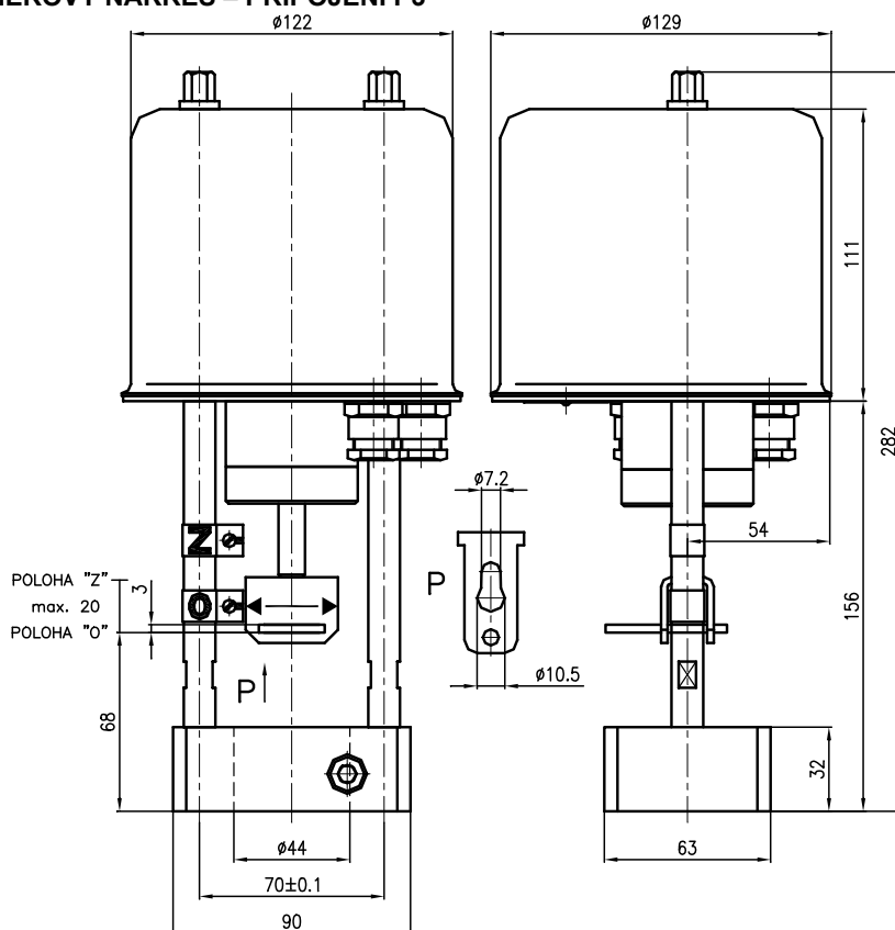
OBRÁZEK 2 - ROZMĚROVÝ NÁKRES – PŘIPOJENÍ P3
