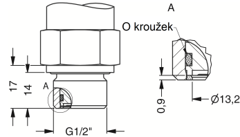
G1/2" DIN 3852 s čelním mečícím článkem
