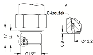
G1/2" DIN 3852 s čelní membránou 4
