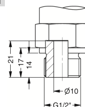
G1/2" DIN 3852 otevřený vstup
