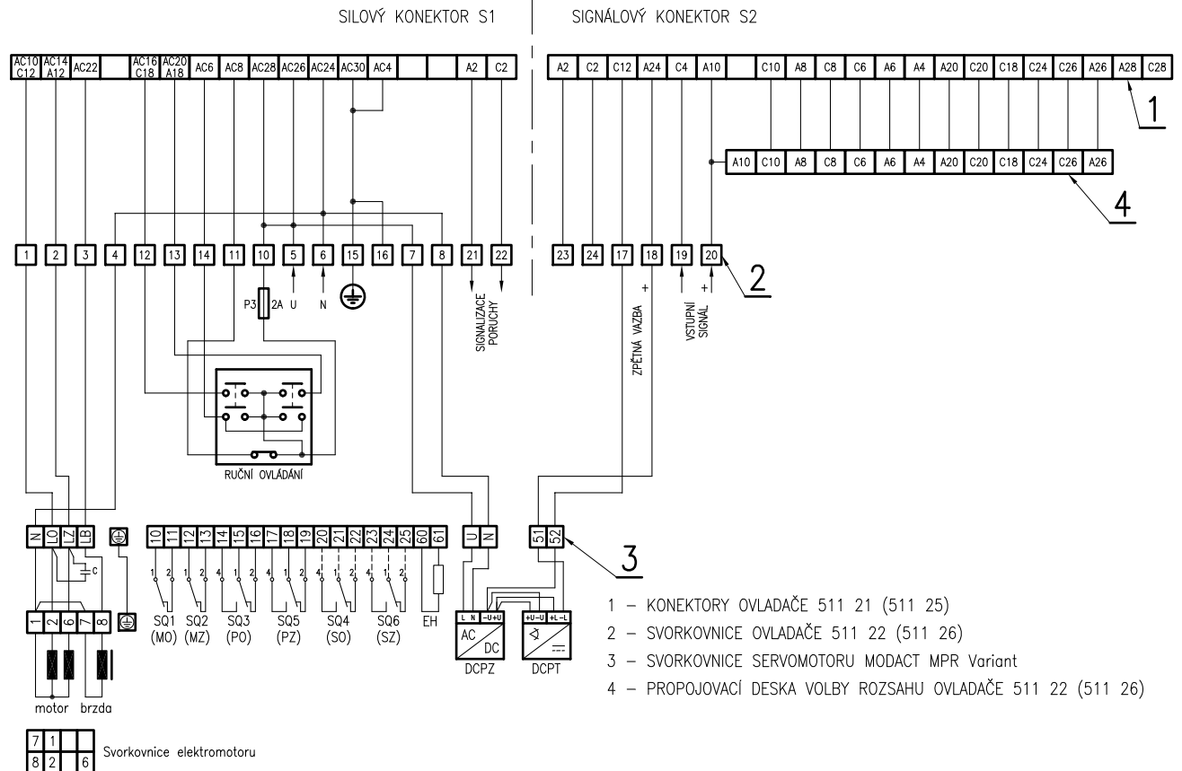
OBRÁZEK 5 - SCHÉMA PŘIPOJENÍ OVLADAČŮ SE SERVO MOTOREM V PROVEDENÍ "SVORKOVNICE"
