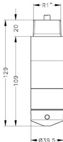
LMK 382 se závitem R1" pro montáž nerezové pružné trubky
