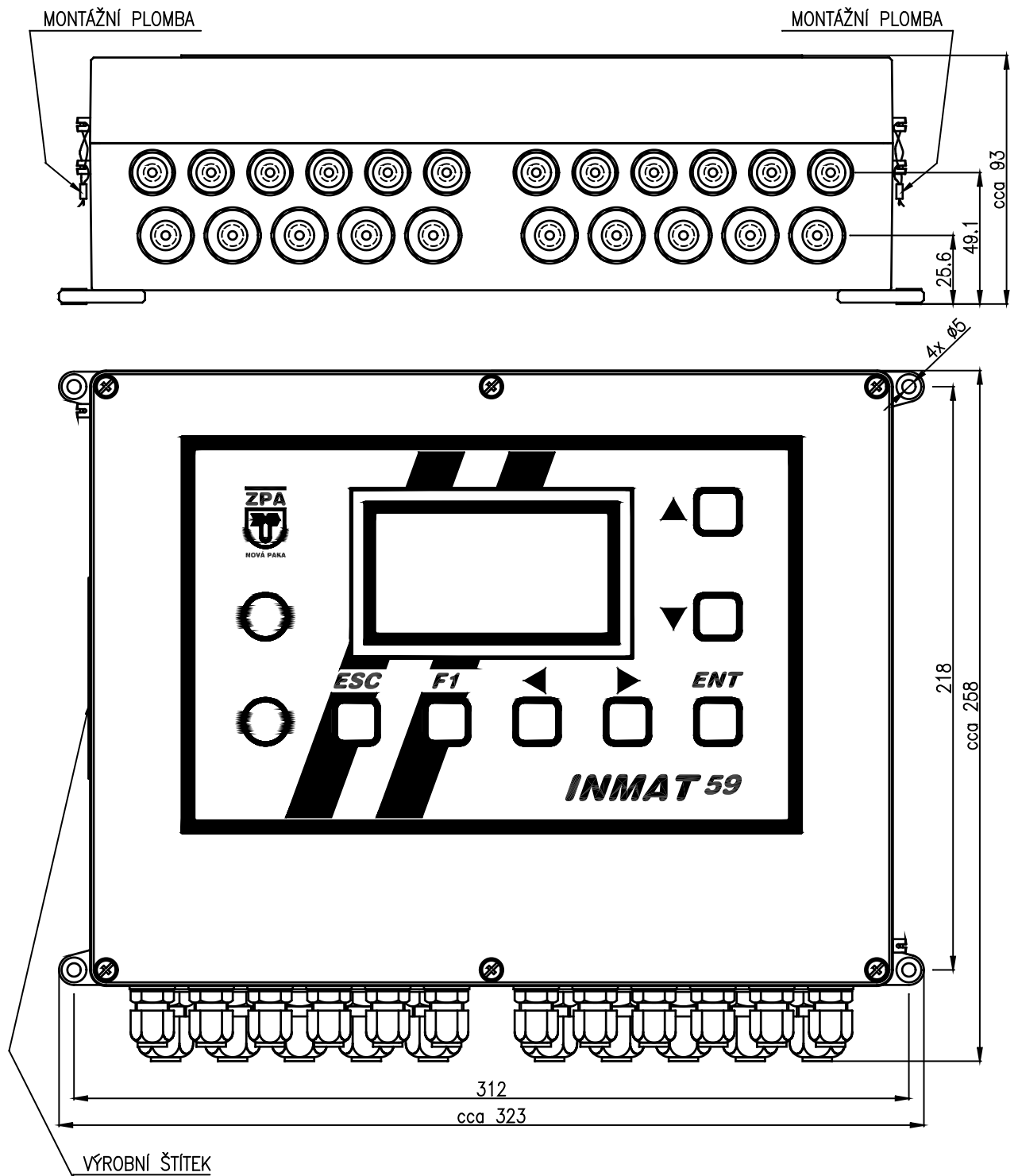
OBRÁZEK 1 - ROZMĚROVÝ NÁKRES
