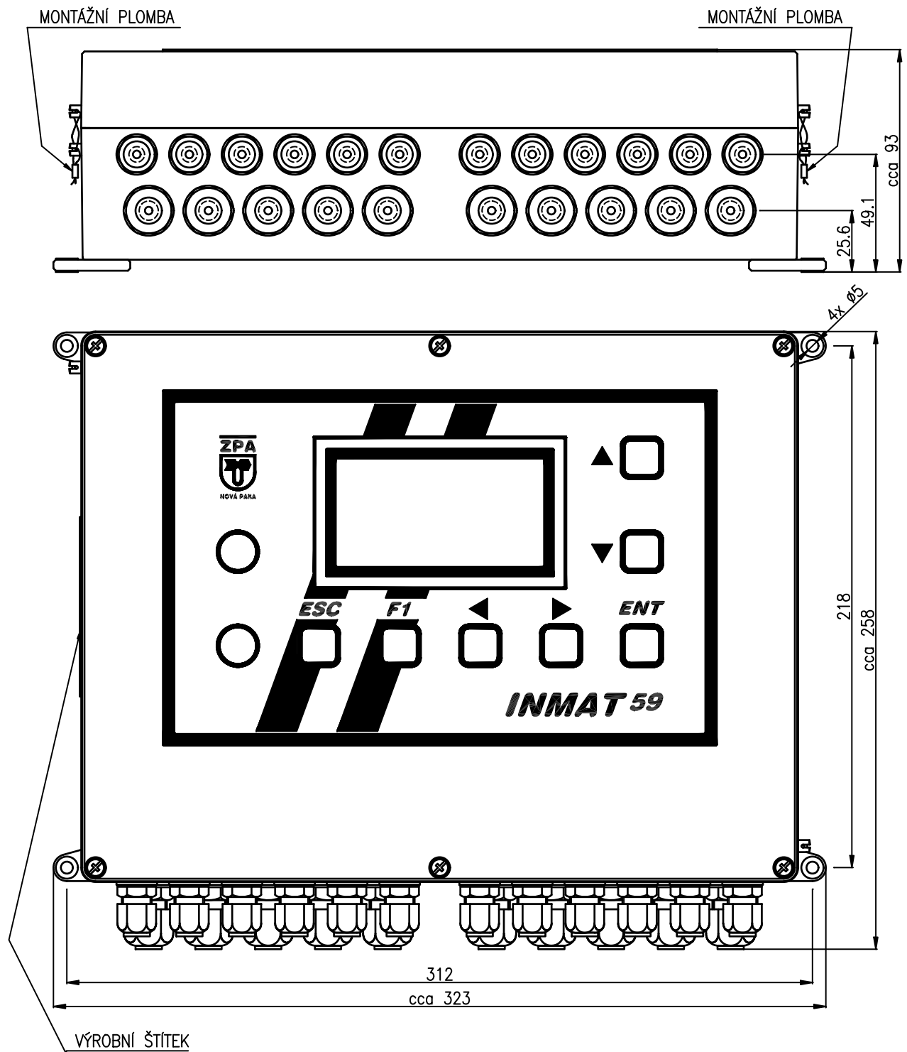
OBRÁZEK 1 - ROZMĚROVÝ NÁKRES
