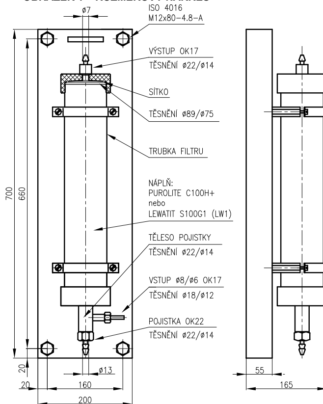
OBRÁZEK 1 – ROZMĚROVÝ NÁKRES
