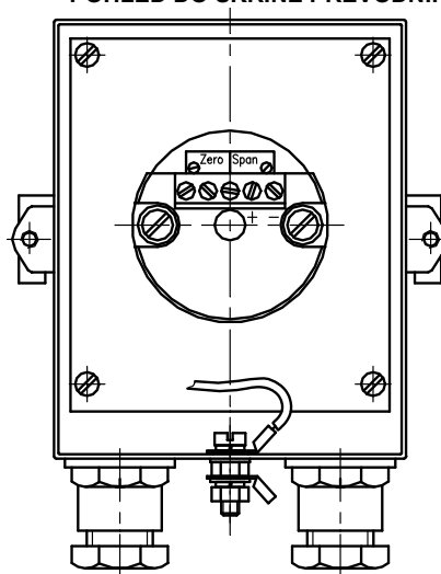
OBRÁZEK 2 - ROZMĚROVÝ NÁKRES A SCHÉMA ZAPOJENÍ PŘIPOJOVACÍ SVORKOVNICE
