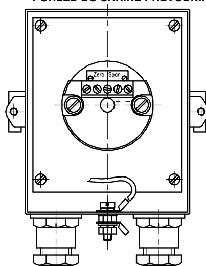
POHLED DO SKŘÍŇE PŘEVODNÍKU
