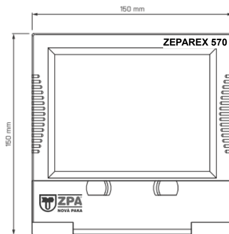
OBRÁZEK 3 – ROZMĚROVÝ NÁKRES
