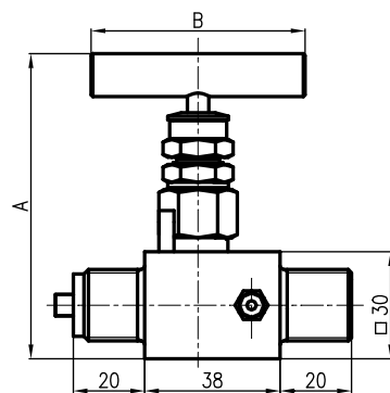
OBRAZEK 6 - TLAKOMĚROVÝ ZKUŠEBNÍ VENTIL S UZAVÍRÁNÍM KONTROLNÍHO ODBĚRU VENTILEM 967 52 31 33, 967 52 31 39, 967 52 35 33 A 967 52 35 39, rozměrový náčrtes, schéma, použití
