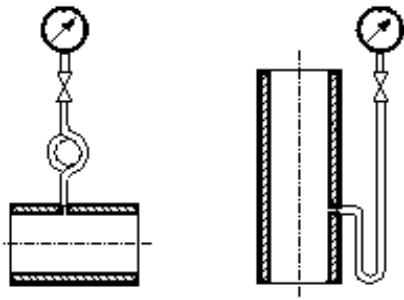
Obrázek 1 - Kondenzační smyčky pro vodorovné a svislé potrubí
