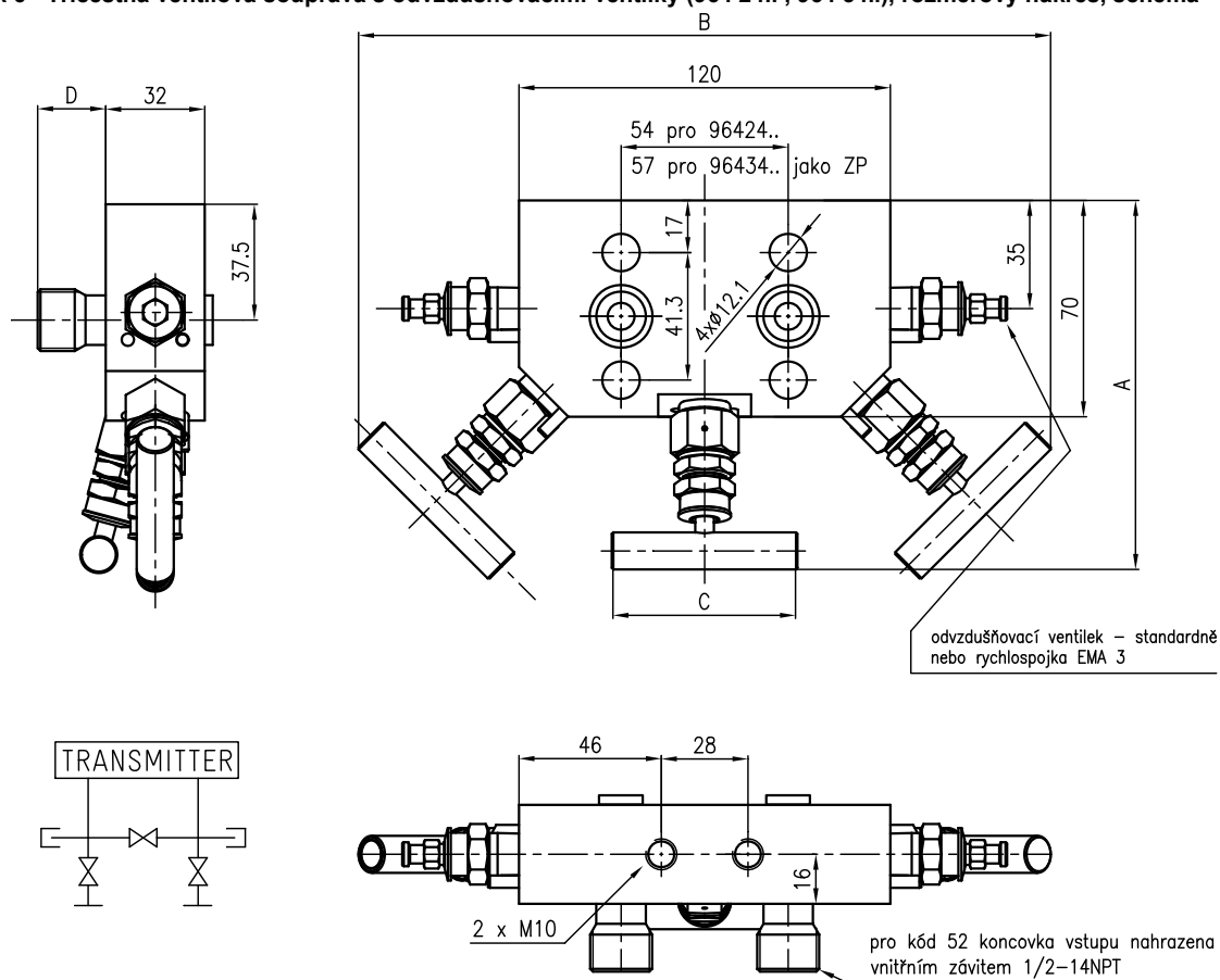
Obrázek 6 - Třicečná ventilová souprava s odvzdušňovacími ventilkami (964 24.. , 964 34..), rozměrový náčrtek, schéma
