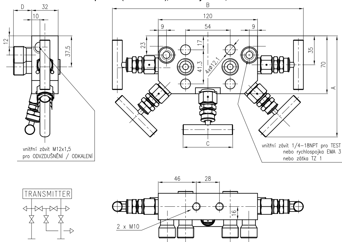
Obrázek 13 - Pěticestná ventilová souprava (964 25.. AS21), rozměrový náčrtek, schéma
