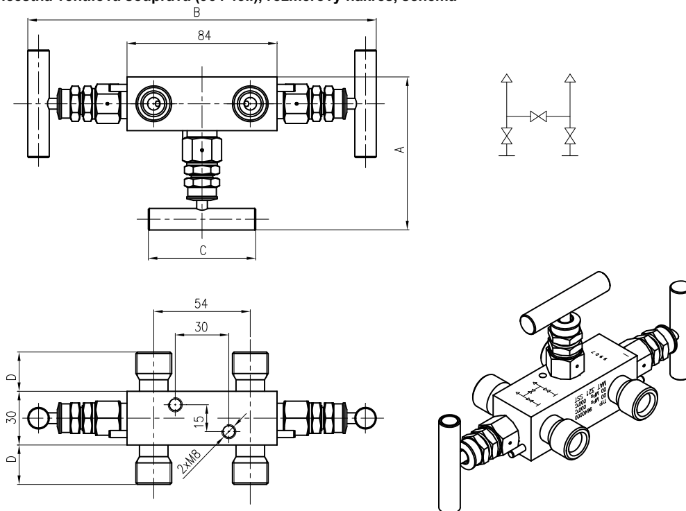
Obrázek 5 - Třicečná ventilová souprava (964 43..), rozměrový náčrtek, schéma
