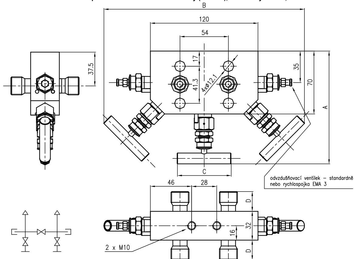
Obrázek 7 - Třicestná ventilová souprava s odvzdušňovacími ventilky (964 44..), rozměrový náčrtek, schéma
