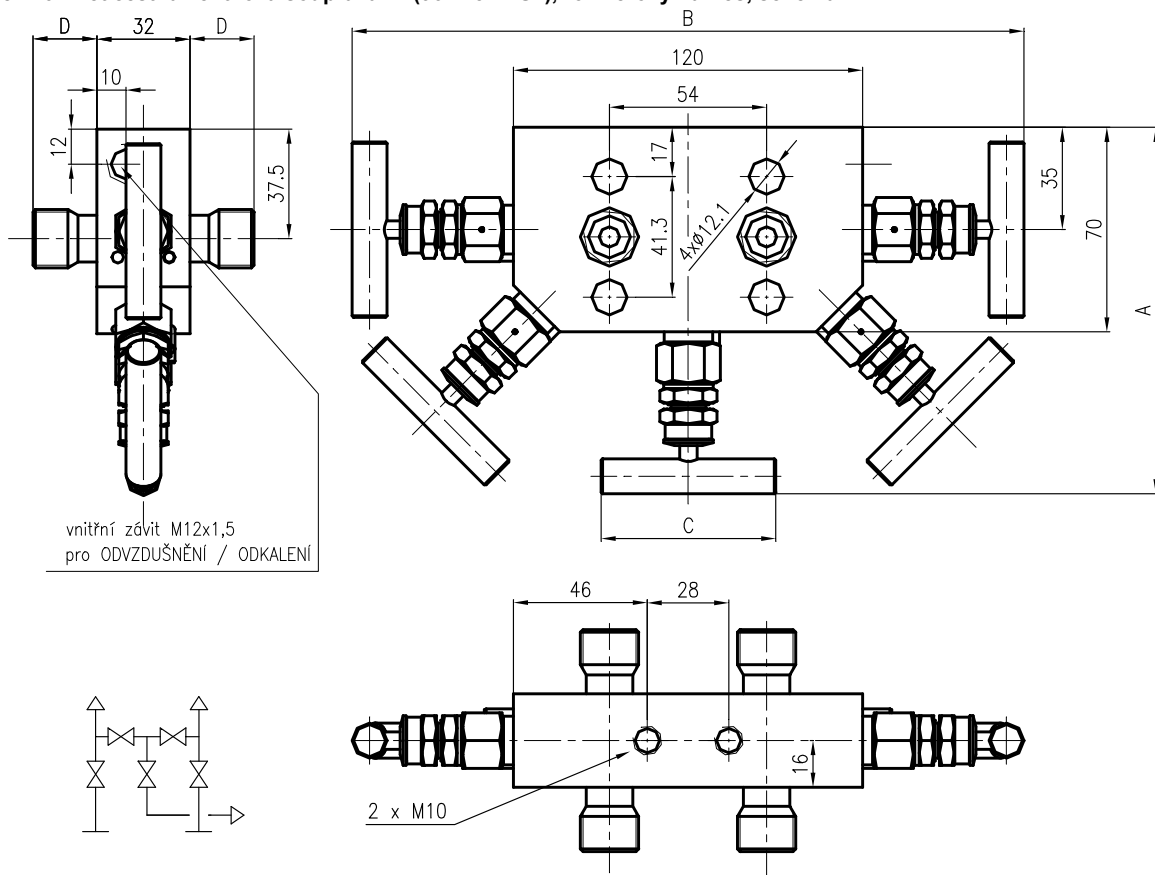
Obrázek 16 - Pěticestná ventilová souprava (964 45.. AS2), rozměrový náčrtek, schéma
