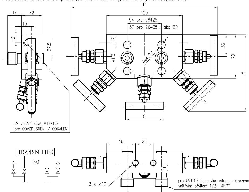
Obrázek 8 - Pěticestná ventilová souprava (964 25.. , 964 35..), rozměrový náčrtek, schéma
