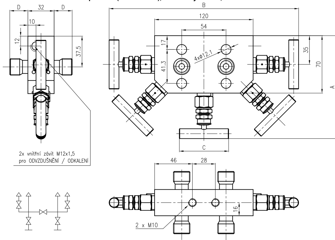
Obrázek 15 - Pěticestná ventilová souprava (964 45.. AS1), rozměrový náčrtek, schéma
