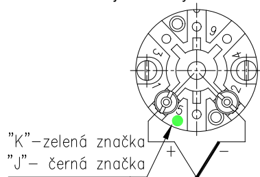
OBRÁZEK 4 - SCHÉMA ZAPOJENÍ SNÍMAČŮ TEPLoty
