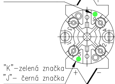
OBRÁZEK 5 - PŘÍKLAD PROVOZNÍHO ZAPOJENÍ SNÍMAČE TEPLoty S PŘEVODNÍKEM VE SMYČCE 4 - 20 mA
