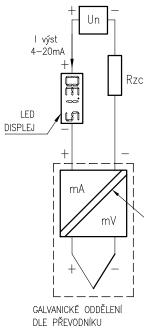
OBRÁZEK 5 - PŘÍKLAD PROVOZNÍHO ZAPOJENÍ SNÍMAČE TEPLoty S PŘEVODNÍKEM VE SMYČCE 4 - 20 mA
