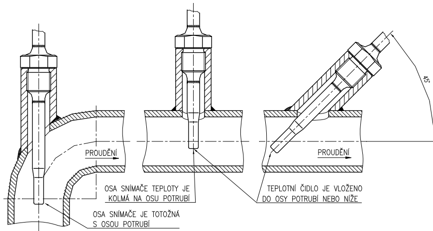
OBRÁZEK 1 - PŘÍKLADY MONTÁŽE PŘÍMÝCH A ŠIKMÝCH NÁVARKŮ DLE ČSN EN 1434-2
